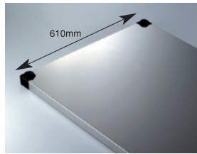
奥行きが610mmのボードは長さが1220mm以上になると補強が2本入ります
