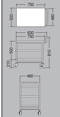
弁慶キッチンワゴン K-3
