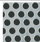
穴径 φ3mm 開孔率 40%
