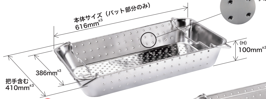
NEW ●18-8 水切運搬バット 100
